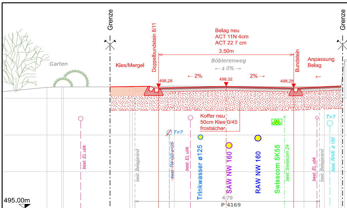
Sanierung Böblereyweg – Normalprofil Strasse und Lage der Werkleitungen östlichen Bereich
